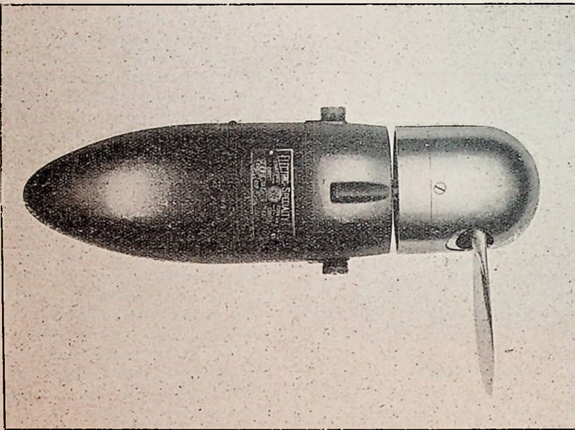
Fig. 3. De luchtschroef van het generatortje heeft maar één blad, hetgeen de automatische regeling van den hoek, waarouder het blad zich voor verschillende snelheden instelt, eenvoudiger maakt.
